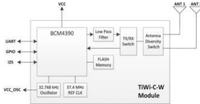
Fig.3: Wifi Module
