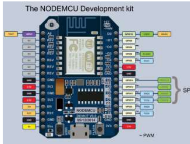
Fig.2: ESP module[3]
